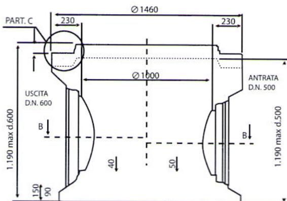
Schéma fond de regard
